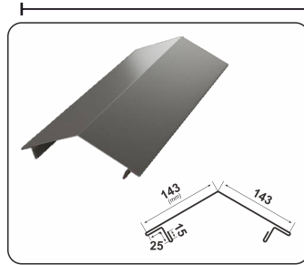
COAMĂ RETRO
