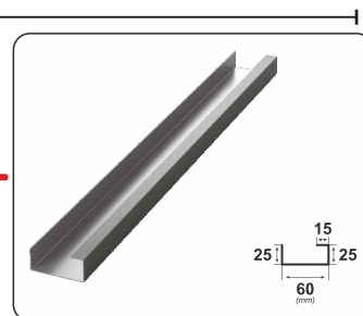
SUPORT COAMĂ
