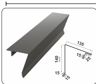
SEMICOAMĂ RETRO
