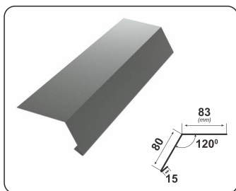
BORDURĂ STREĂȘINĂ
