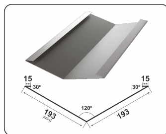
DOLIE RETRO
