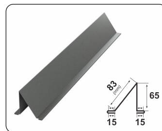
OPRITOR ZAPADĂ
