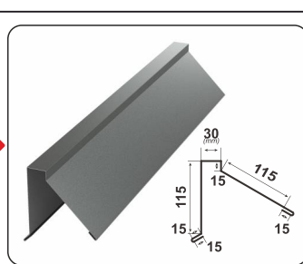
SEMICOAMĂ UNGHIULARĂ
